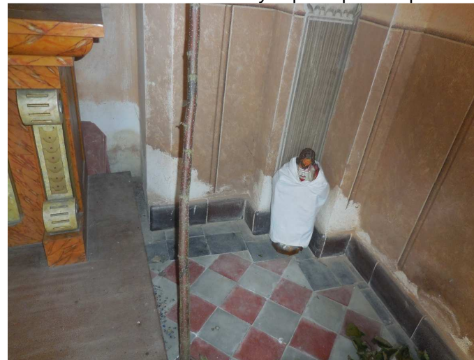
Poškození omítek nad vnitřním keramickým soklem
